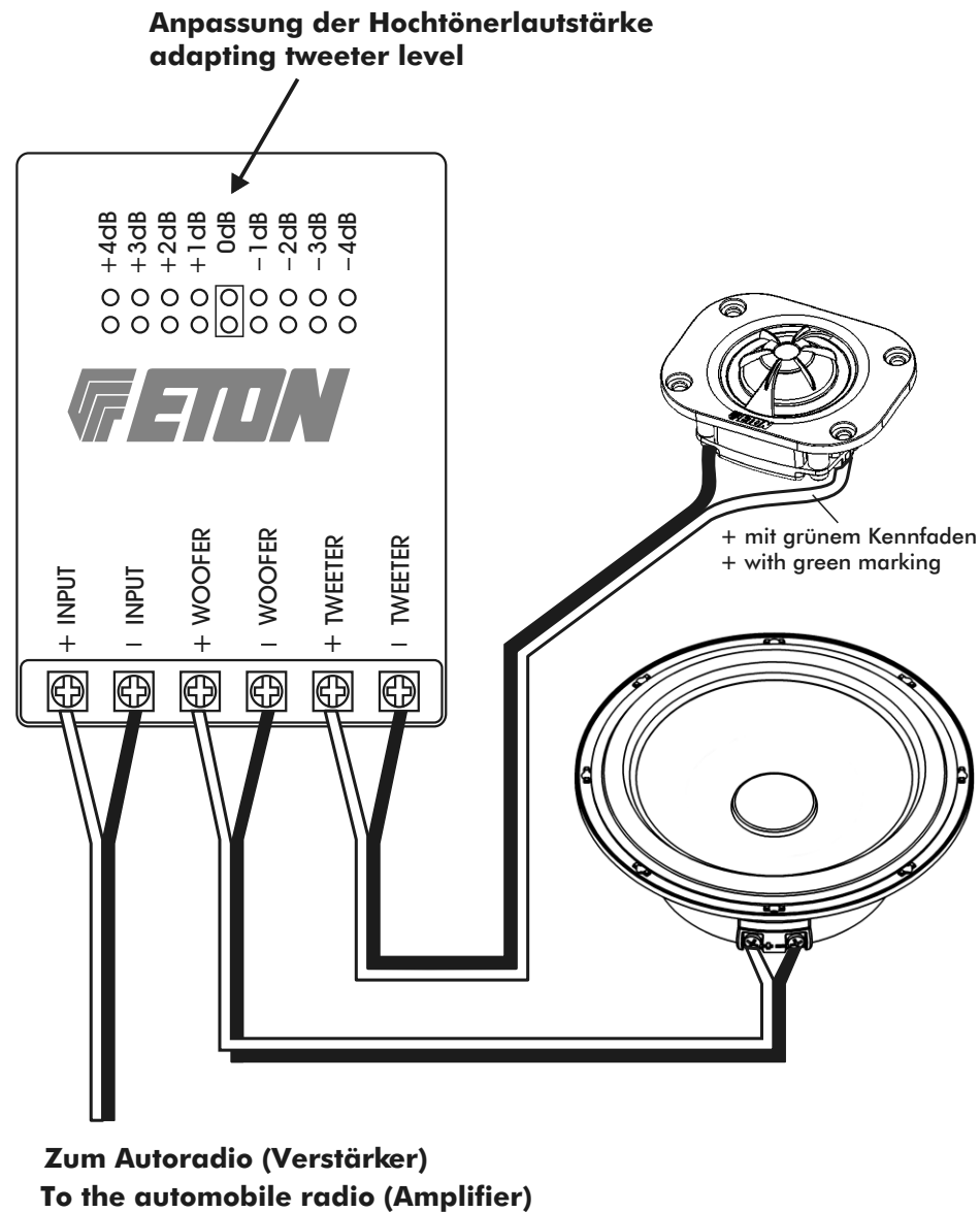
Anschlußplan für Weiche Wiring diagram crossover
